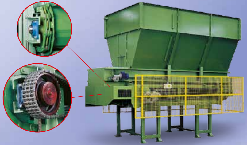
Hopper Trichter
